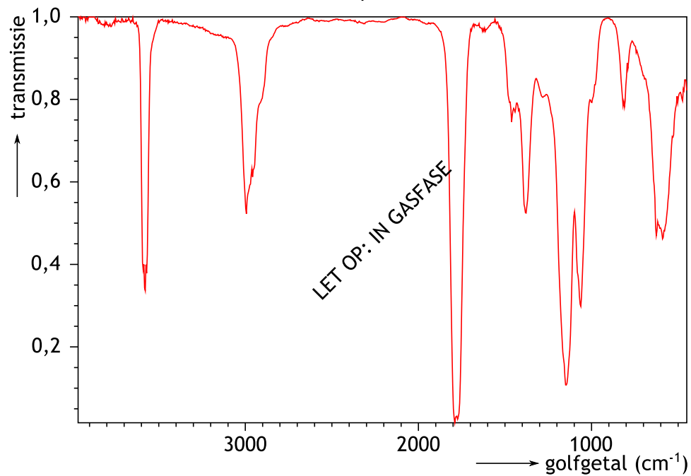
IR-spectrum
