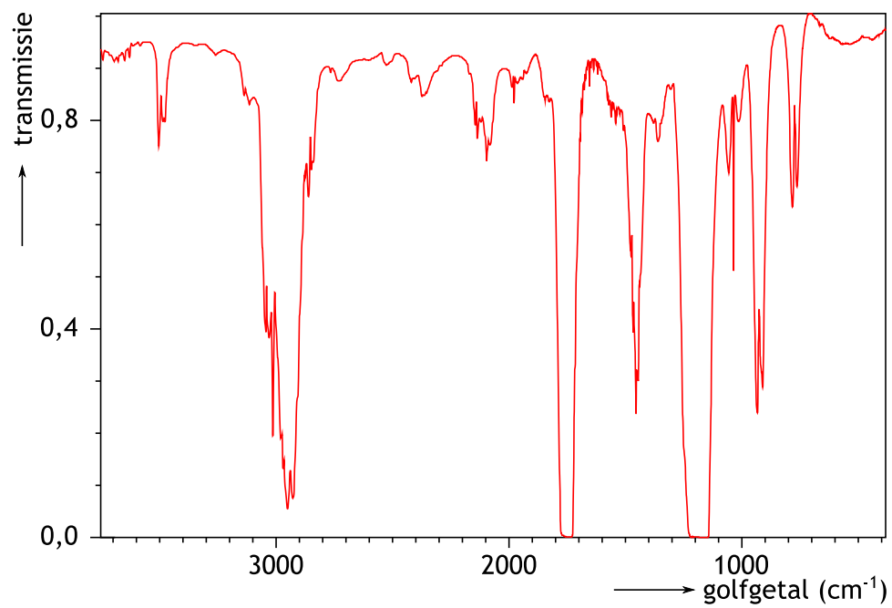
IR-spectrum
