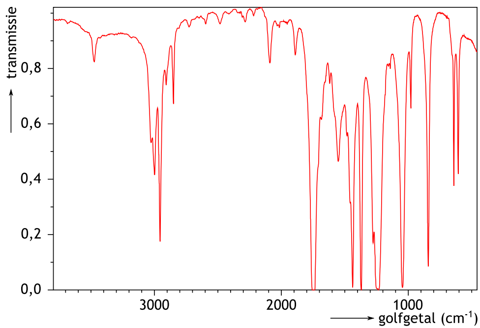
IR-spectrum
